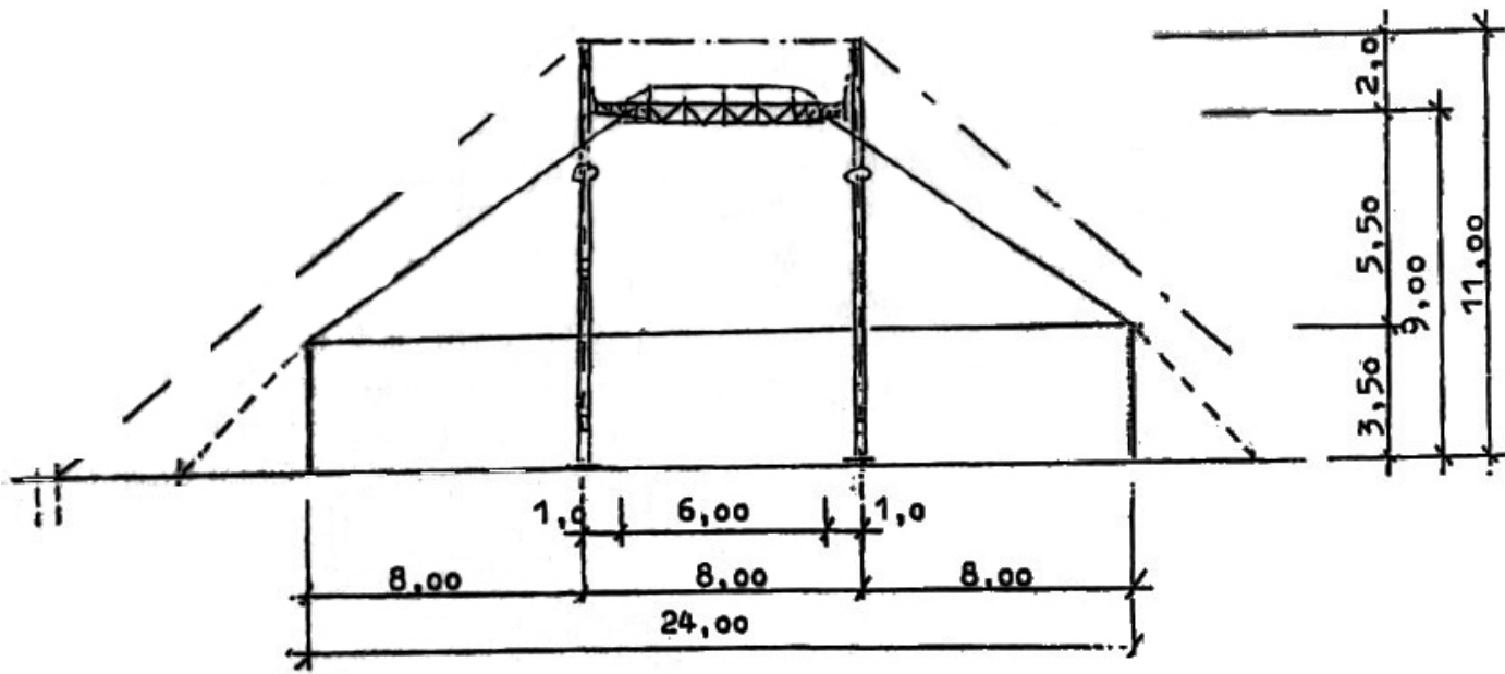
Längsschnitt M 1 : 200
